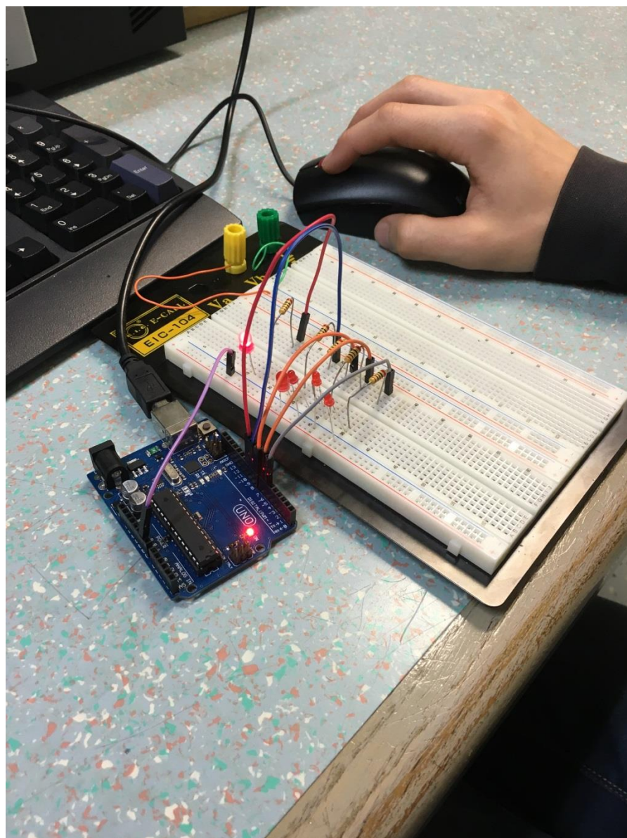
Plošča ArduinoUNO.
